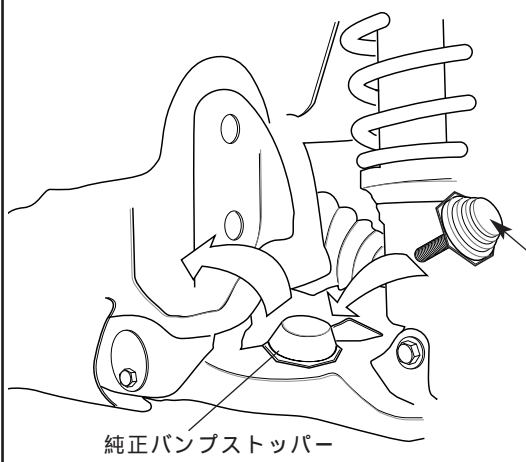
図2 リヤバンプストッパー延長ブラケットの取付
