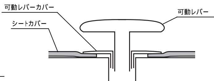
可動レバー部断面図
